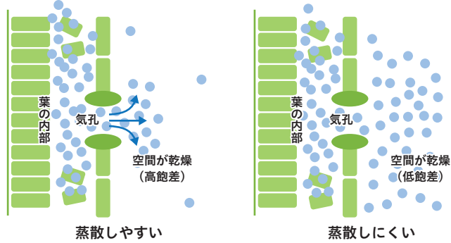
■第2図 飽差による蒸散への影響と制御機器 葉の周辺の飽差と蒸散
