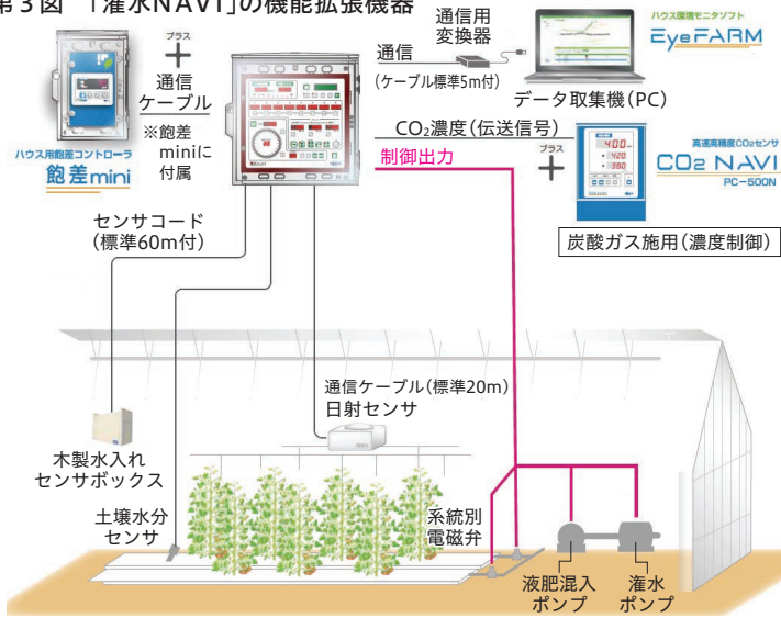
■第3図 「灌水NAVI」の機能拡張機器
